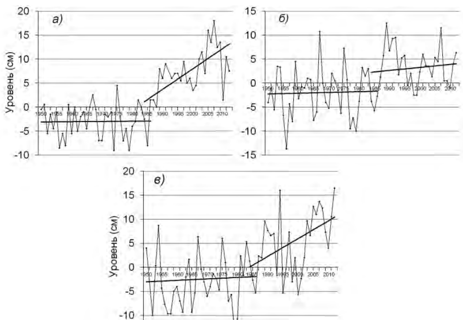
Рис. 3.26. Аномалии среднегодового уровня, осредненные по районам арктических морей. а – юго-запад Карского моря; б – восток Карского моря; в – Новосибирские острова. Прямыми линиями показаны линейные тренды.
