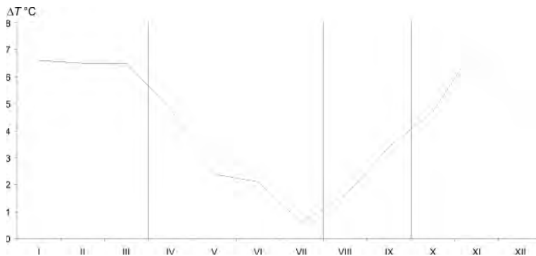
Рис. 1.9. Годовой ход среднемесячных значений аномалии температуры воздуха (°C) в широтном поясе 70–85° с.ш. в 2012 г.
