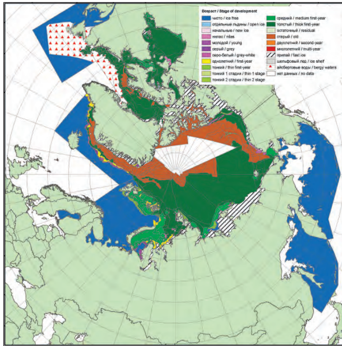
Рис. 2.14. Обзорная ледовая карта СЛЮ за 15–16 мая 2012 г., составленная на основе ледового анализа ААНИИ, КЛС и НЛЦ США.
