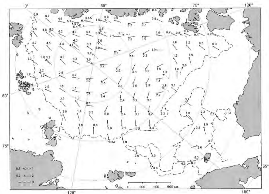
Рис. 2.26. Поле скорости результирующего дрейфа льда (км/сут) за август 2012 г. Усл. обозначения см. рис. 2.23.
