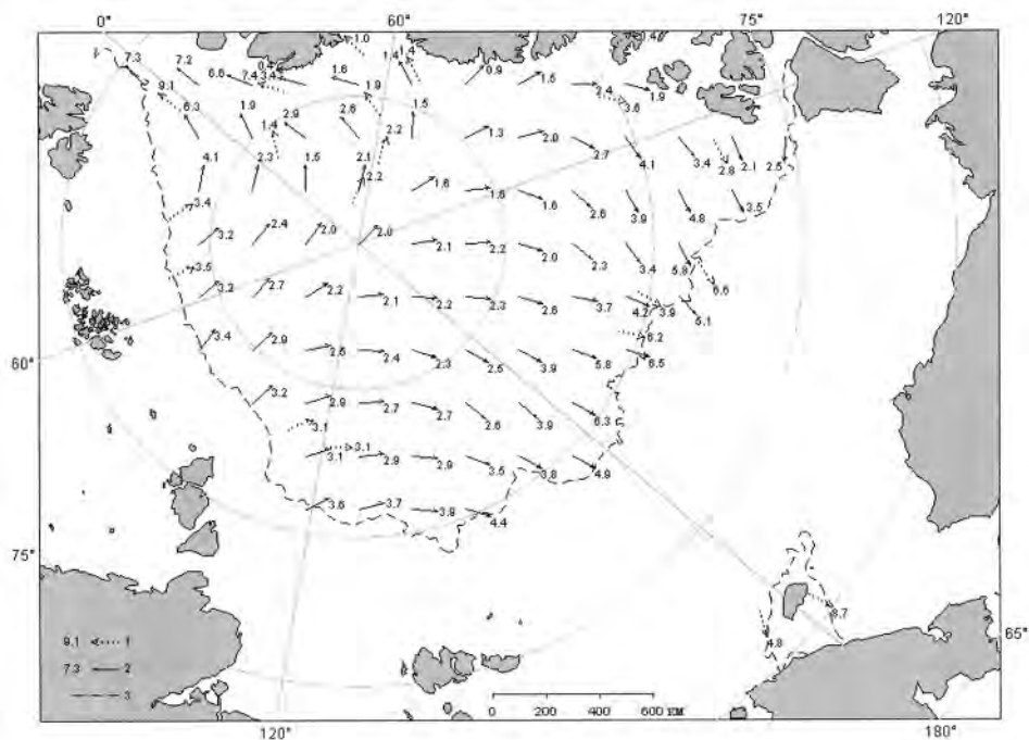
Рис. 2.29. Поле скорости результирующего дрейфа льда (км/сут) за сентябрь 2012 г. Усл. обозначения см. рис. 2.23.
