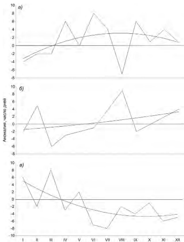
Рис. 1.1. Годовой ход среднемесячных аномалий числа дней с основными формами циркуляции в 2012 г. а – западная форма, б – восточная форма, в – меридиональная форма.
