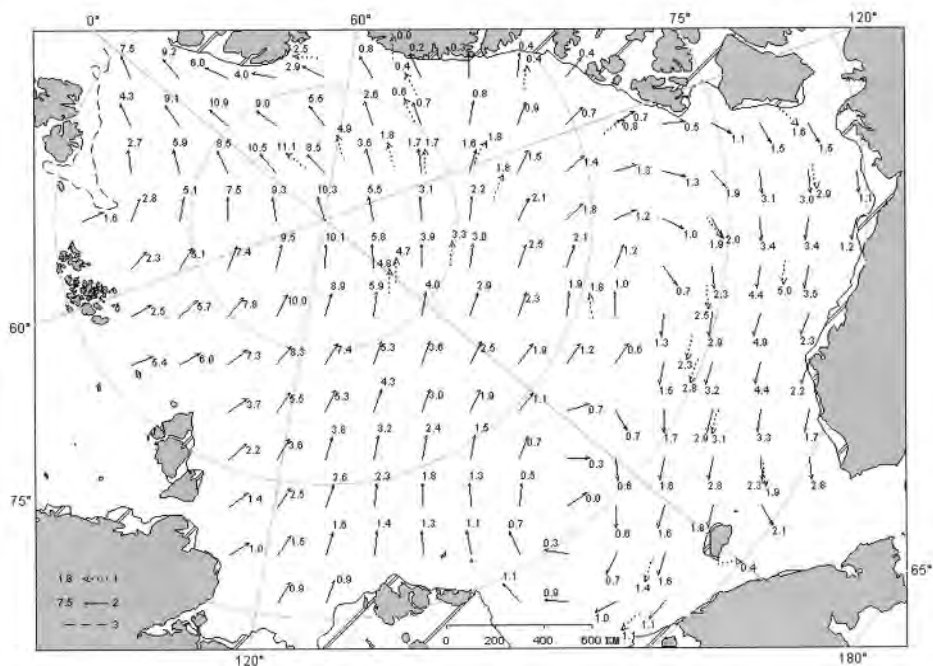
Рис. 2.6. Поле скорости результирующего дрейфа льда (км/сут) в феврале 2012 г. Усл. обозначения см. рис. 2.3.
