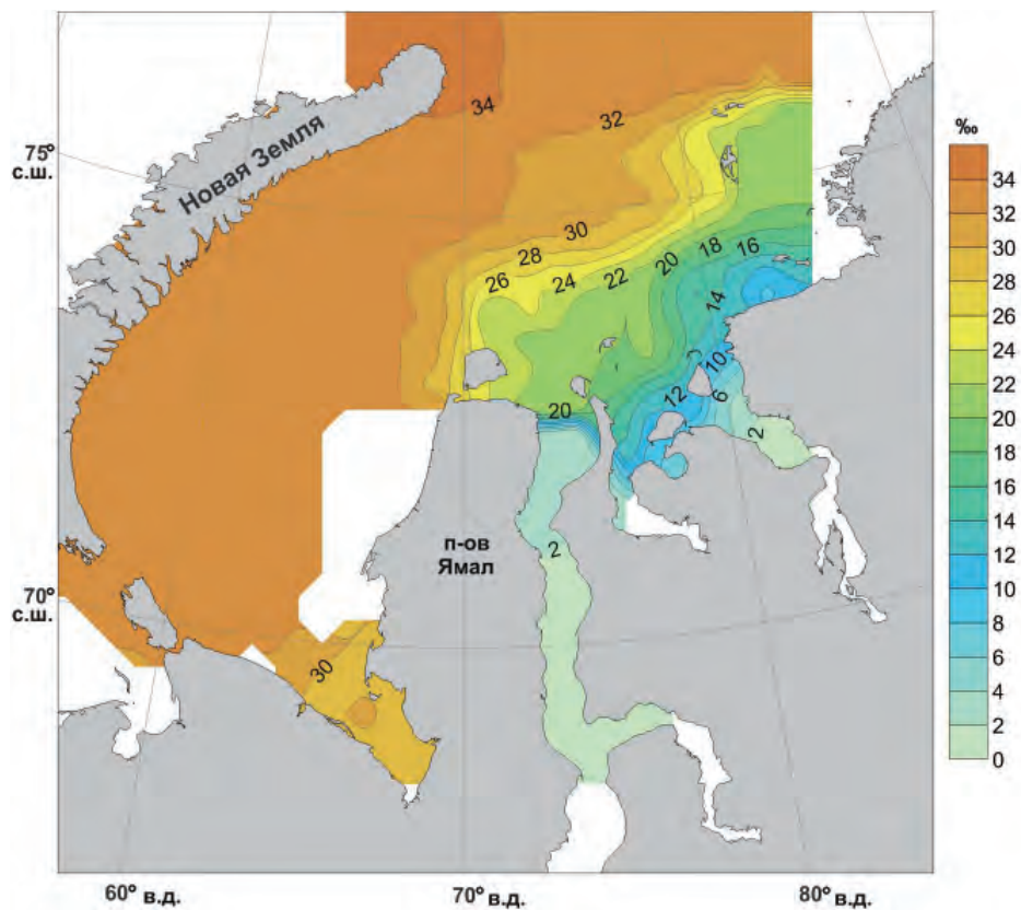
Рис. 3.16. Распределение поверхностной солёности (‰) в Карском море по результатам экспедиции «Ямал – Арктика 2012».
