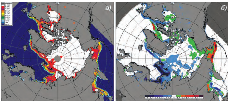
Рис. 2.4. Медианное распределение плотности льда в январе 2012 г. (а) и ее разность относительно медианного распределения за тот же месяц за период 1979–2012 гг. (б) на основе расчетов по данным SSMR-SSM/I, алгоритм NASATEAM.
