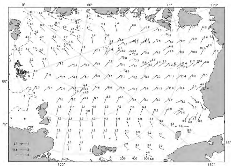
Рис. 2.35. Поле скорости результирующего дрейфа льда (км/сут) за ноябрь 2012 г. Усл. обозначения см. рис. 2.32.
