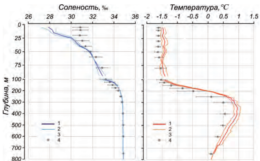
Рис. 3.6. Вертикальное распределение солёности и температуры воды по результатам измерений экспедиции «Арктика-2012» в районе хребта Менделеева в третьем квартале 2012 г.
