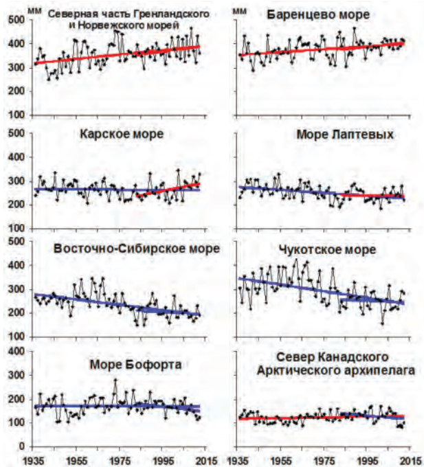
Рис. 1.14. Временные ряды годовых сумм осадков.
