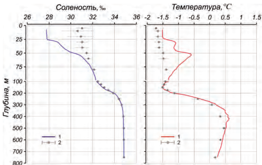
Рис. 3.4. Характерное вертикальное распределение солёности и температуры воды по результатам STD-зондирования в точке с координатами 75,27° с.ш., 133,22° з.д., выполненного 12 марта 2012 г. бумом ИТР-41.
