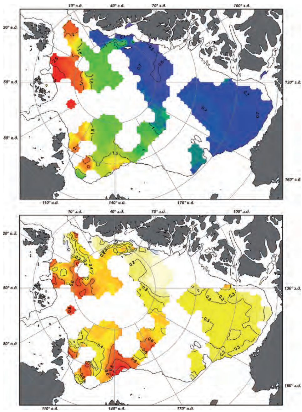
Рис. 3.14. Пространственное распределение температуры ядра АВ (°C) в 2012 г. (вверху) и ее аномалий (°C) по отношению к среднему значению за период 1950–1994 гг. (внизу).
