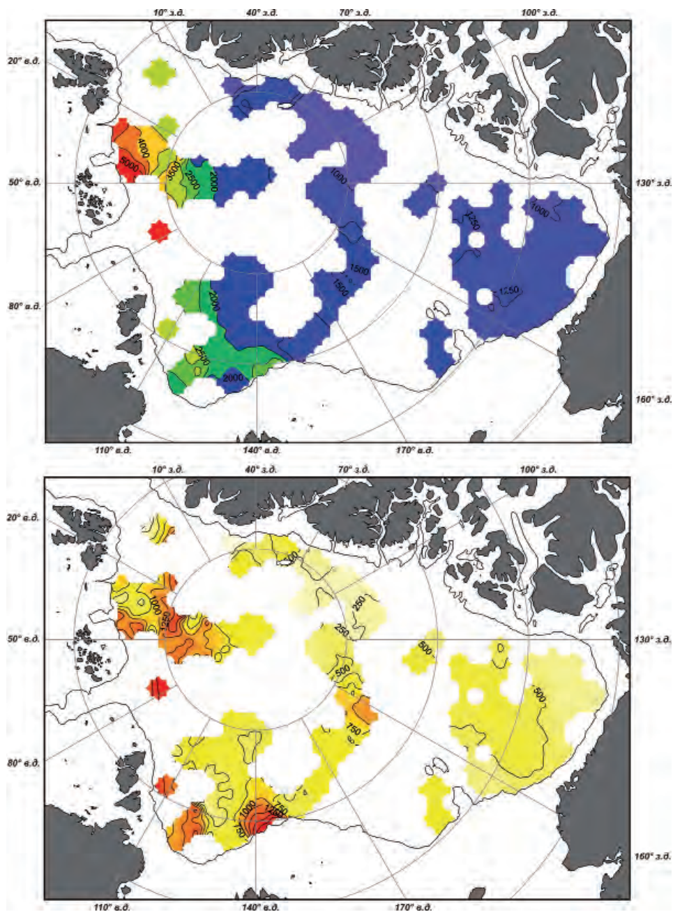
Рис. 3.15. Пространственное распределение теплосодержания (МДж/м 2 ) слоя АВ в 2012 г. (вверху) и его аномалий (МДж/м 2 ) по отношению к среднему значению за период 1950–1994 гг. (внизу).
