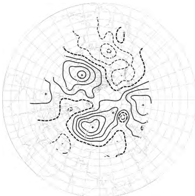
Рис. 1.5. Поле средней аномалии приземного давления (гПа) за период январь–декабрь 2012 г.
