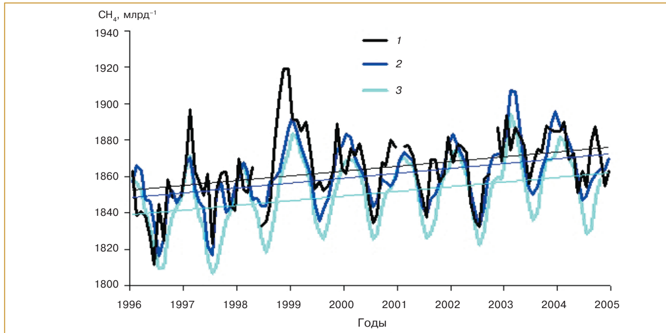
Рис. 4.3. Временной ход концентрации метана на станции Териберка (1) за период 1996–2005 гг. (Парамонова и др., 2001). Для сравнения приводятся изменения концентрации \text{CH}_4 на станциях Барроу (США) (2) и Алерт (Канада) (3). Прямые — линейные тренды.
