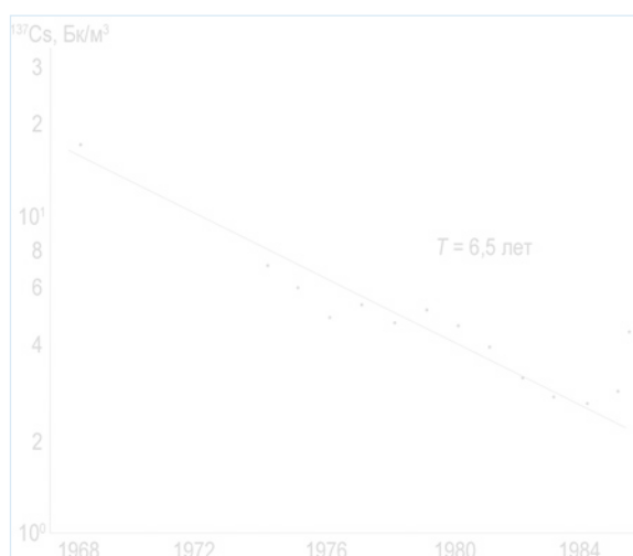
Рис. 2. Динамика уровней ^{137}\text{Cs} в воде озер и рек Восточной Финляндии (1968–1985). T — полупериод очищения озерно-речных систем
