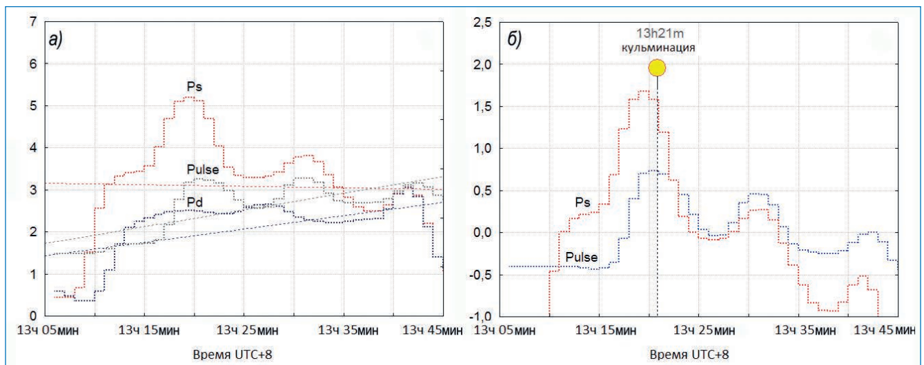
Рис. 2. Распределения показателей артериального давления (Ps, Pd) и артериального пульса (Pulse) человека в полуденном интервале 13 ч 00 мин – 13 ч 45 мин за период с 22.01.2017 года по 18.04.2017 года. НИС «Ледовая база Мыс Баранова».
