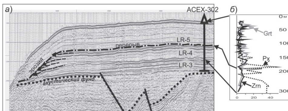
Рис. 3. Фрагмент сейсмического профиля AWI-91090 [Jokat, 2005], проходящий через скважину АСЕХ-302 (а), и кривые содержания минералов ТФ (Grt – светло-серая, Zrn – темно-серая, Pх – пунктир) по скважине АСЕХ-302 [по Krylov et al., 2008].
