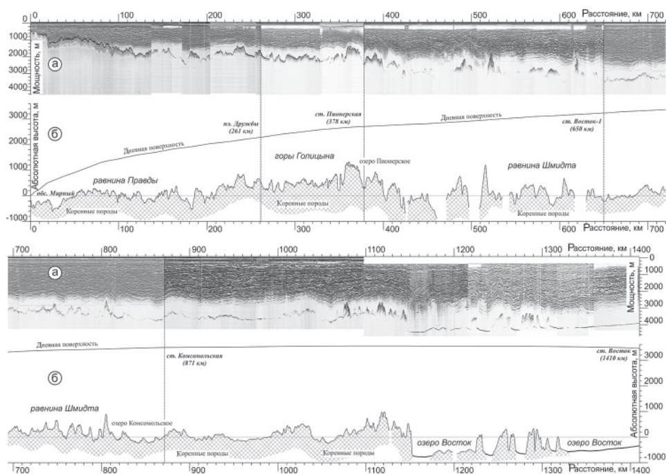
Рис. 2. Временной радиолокационный разрез (а) и разрез ледникового покрова (б) по трассе следования СПГ «Мирный–Восток».
