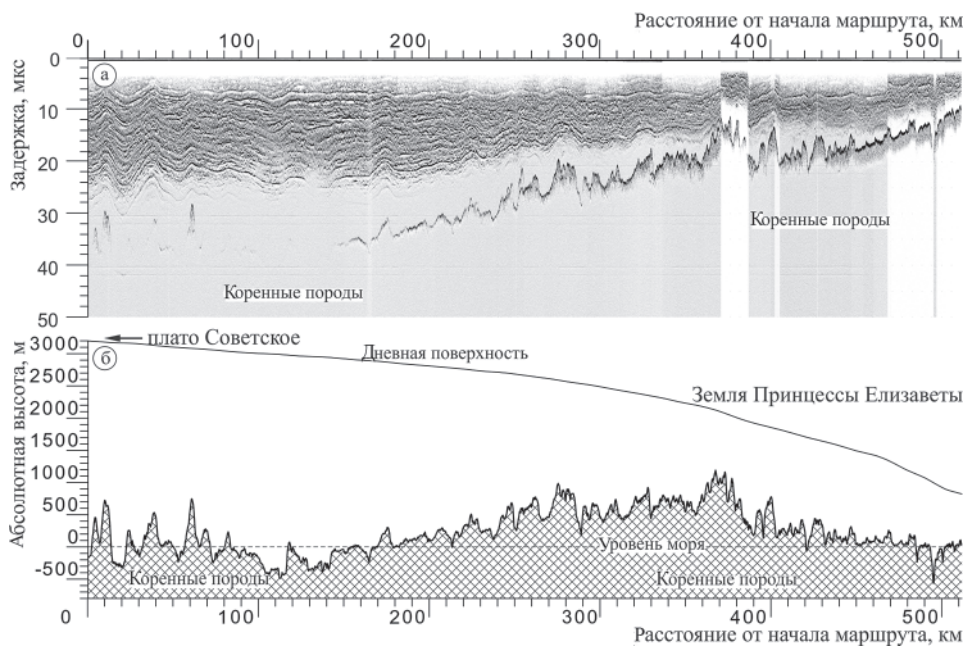
Рис. 3. Временной радиолокационный разрез (а) и разрез ледникового покрова (б) по трассе следования СПГ «Прогресс–Восток».
